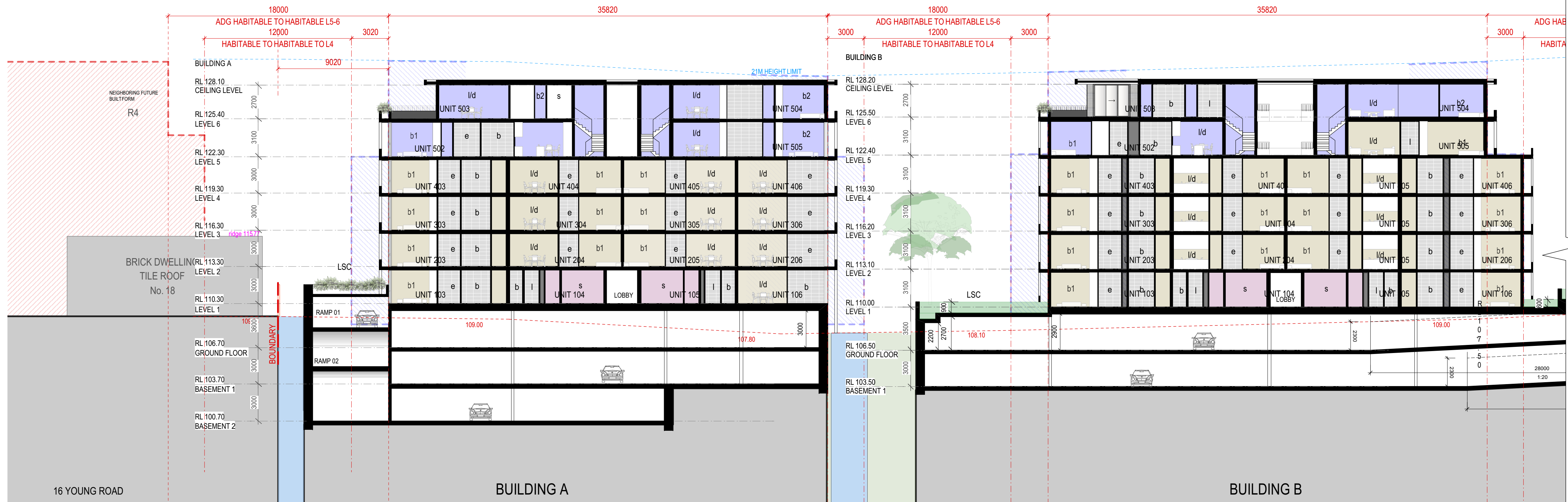
■ SITE SECTION D-D
